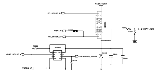
BATTERY CON
